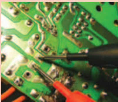
Рис. 3 Измеряем напряжение на выходе фильтра и выходе выпрямителя. Щупы ставим на вход выпаянного выпрямителя. Полярность не имеет значения, так как ток переменный.
